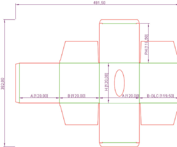
Şekil 10. Karton kutu bıçak izi şeması. Kırmızı çizgiler kesimi, yeşil çizgiler kıvrımı göstermektedir (Hayta, 2015)
