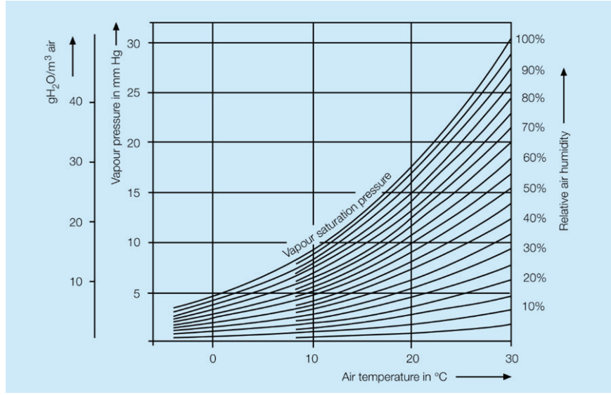
Şekil 4. Sıcaklık ve nem ilişkisi (Sappi, 2025)
