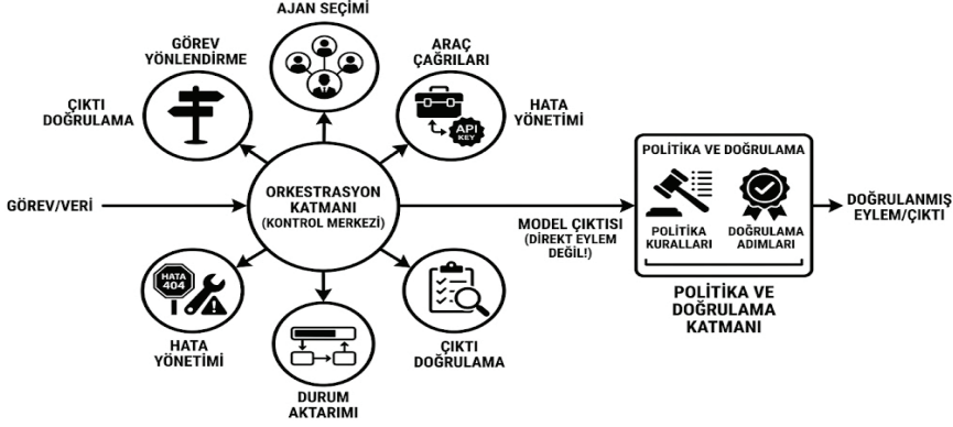
Şekil 2.2: Orkestrasyon katmanı ve kontrol mekanizmaları
