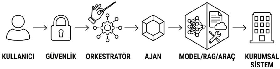
Şekil 5.1: Kurumsal Yapay zekâ orkestrasyonu için referans mimarisi
