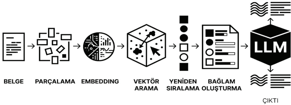
Şekil 2.1: RAG Mimarisi
