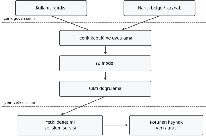
Şekil 1. İçerik akışı ile işlem yetkisinin ayrıldığı örnek güven sınırları
