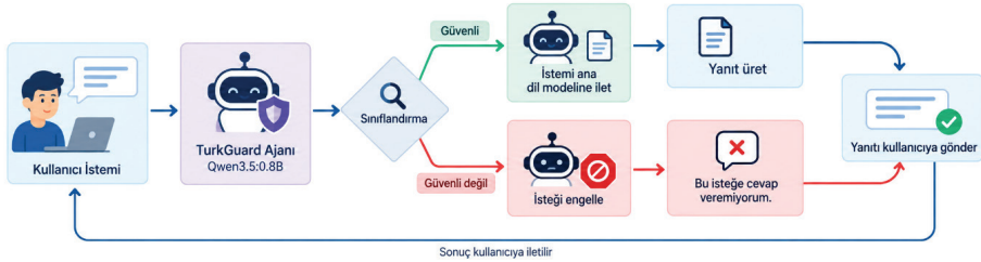
Şekil 3. Korumucu Ajan Mimarisi (Aytaş vd., 2026b)
