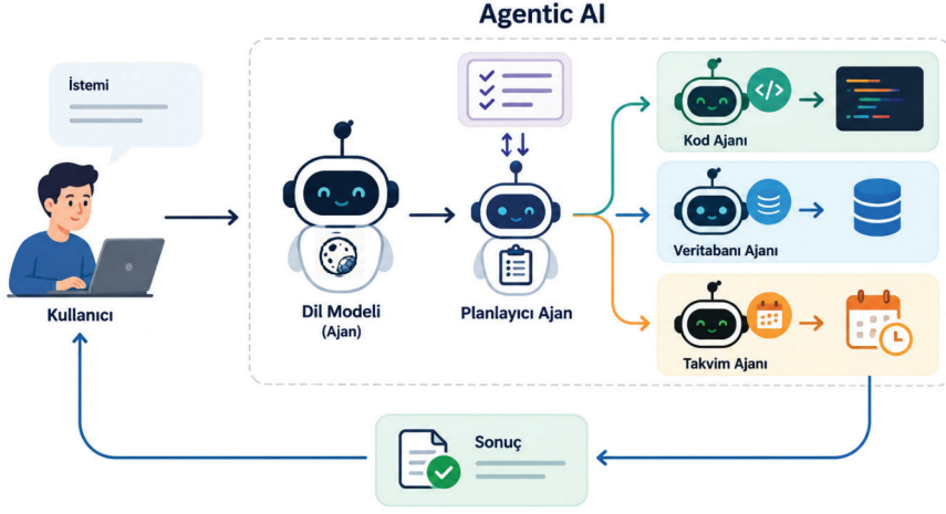
Şekil 2. Ajan Mimarisi
