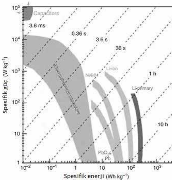
Şekil 1. Ragone grafiği.
