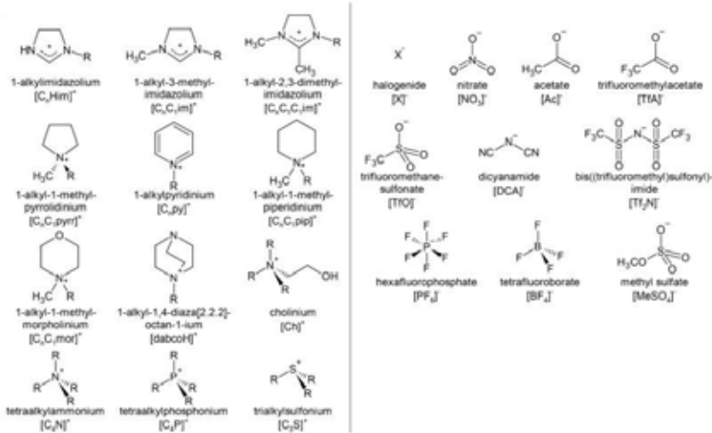
Şekil 5. İyonik sıvıların sentezlenmesinde sık kullanılan katyon (solda) ve anyonlar (sağda) (Plotka-Wasyłka et al., 2020).
