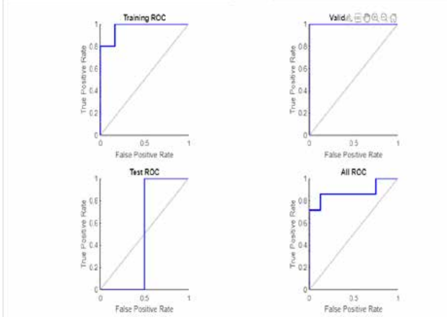
Şekil 5. 2020 Yılı Eğitim, Geçerlilik, Test ve Tümü ROC Eğrileri
